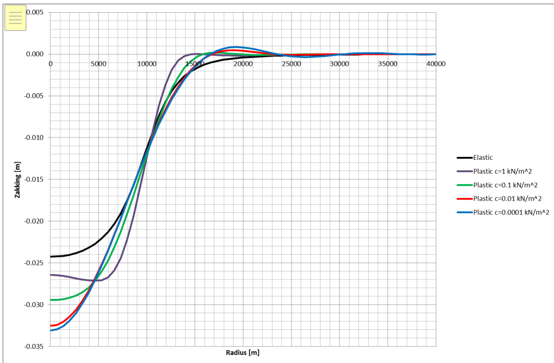
Abbildung 5.1 Auswirkung der zunehmenden Plastizität der Salzsicht auf die Bodensenkung. Die Plastizität nimmt zu, wenn der Kohäsionsparameter gesenkt wird. Die Absenkung in der Mitte der Senkung kann bis zu 35 % höher sein als in der elastischen Berechnung. Der Radius der Senkung wird kleiner.
